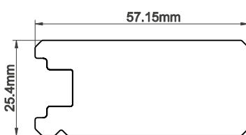
57mm Plain Butt Stile
