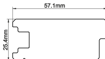
57mm Plain Rebate Stile
