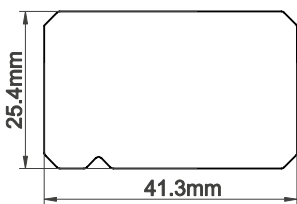
41.3mm Plain Butt Stile
