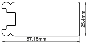
57mm Butt Stile
