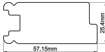
57mm Rebate Stile
